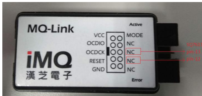
图 8.6 将 MQ-Link Pin6, pin8 對 SQ7617 pin13 與 pin12 连接
