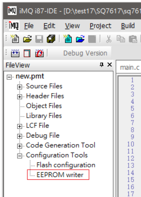
图 6.26 FileView 窗口
